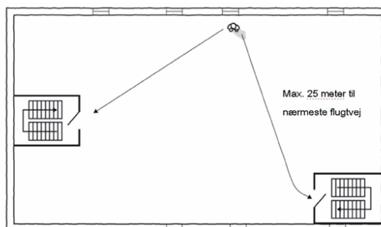
Figur1: Eksempel på lokaler på 1. sal. Hvor der fra underkant af redningsåbningerne (vinduerne) er mere end 2 meter over terræn – og hvorfra der fra lokalerne ikke er 2 helt uafhængige flugtveje I sådanne lokaler er midlertidig overnatninger IKKE tilladt.
