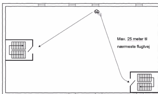
Figur1: Eksempel på lokaler på 1. sal. Hvor der fra underkant af redningsåbningerne (vinduerne) er mere end 2 meter over terræn – og hvorfra der fra lokalene ikke er 2 helt uafhængige flugtveje I sådanne lokaler er midlertidig overnatning IKKE tilladt.
