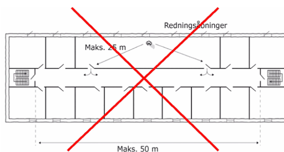
Figur1: Eksempel på lokaler på 1. sal. Hvor der fra underkant af redningsåbningerne (vinduerne) er mere end 2 meter over terræn – og hvorfra der fra lokalene ikke er 2 helt uafhængige flugtveje I sådanne lokaler er midlertidig overnatning IKKE tilladt.
